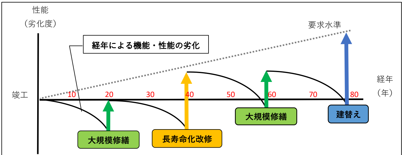
図3-1. 長寿命化のイメージ（鉄筋コンクリート造等で長寿命化を図る場合）
