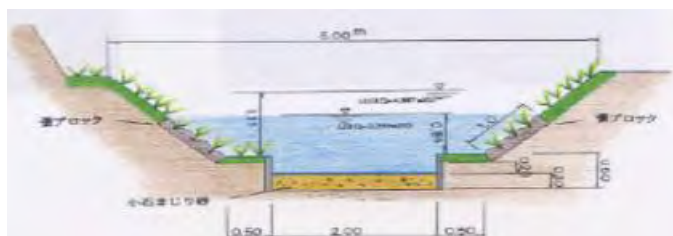
複断面水路
